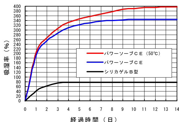
Fig. 2 吸湿速度（25℃, RH90%）
